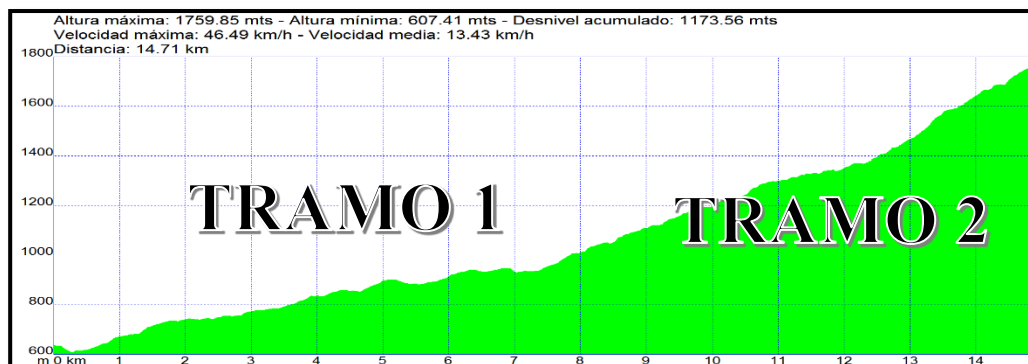
Figura 4. Grafica de la vía de altura en metros con relación distancia en kilómetros, se denota el eje donde se dividirá la vía para realizar el estudio de factibilidad.
